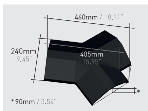
Q123*K | Angular 3 way ridge klinker
