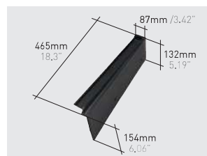
Q116*K | Innova/Vienna right side course klinker
