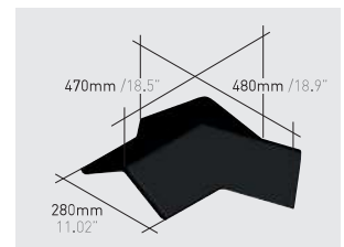
Q111*K | Atica 120° 3 way ridge klinker
